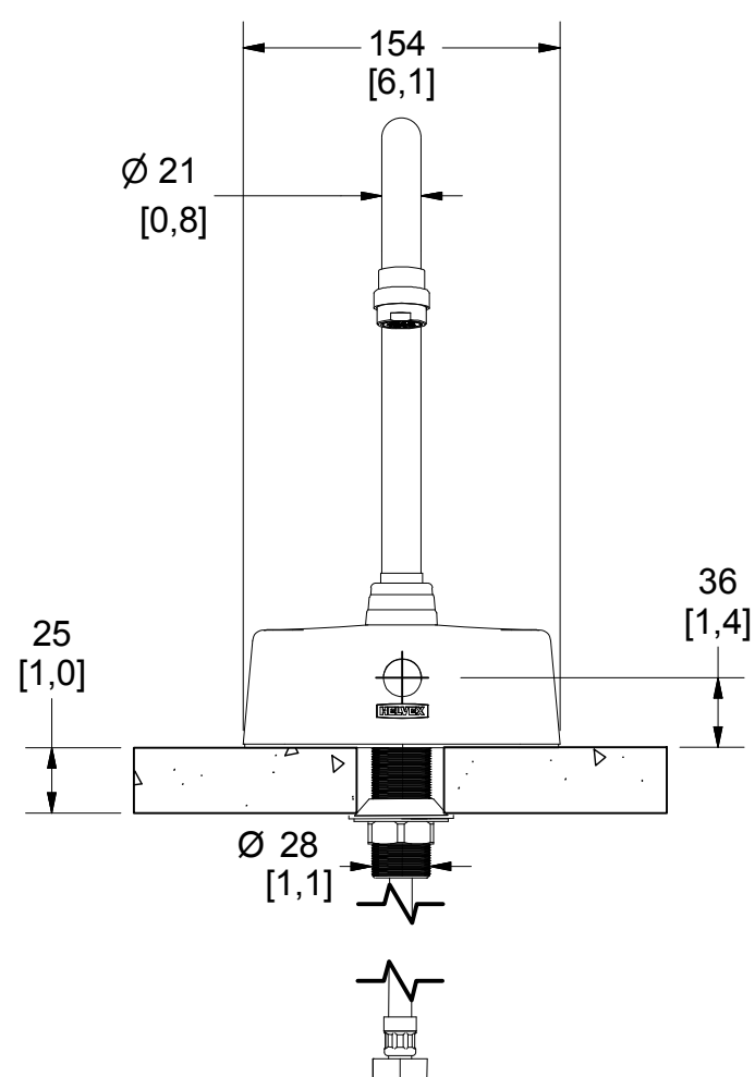
Medidas Referenciales / Estimated Dimensions, Acot. mm [pulg.] / Dim. mm [inch.]
